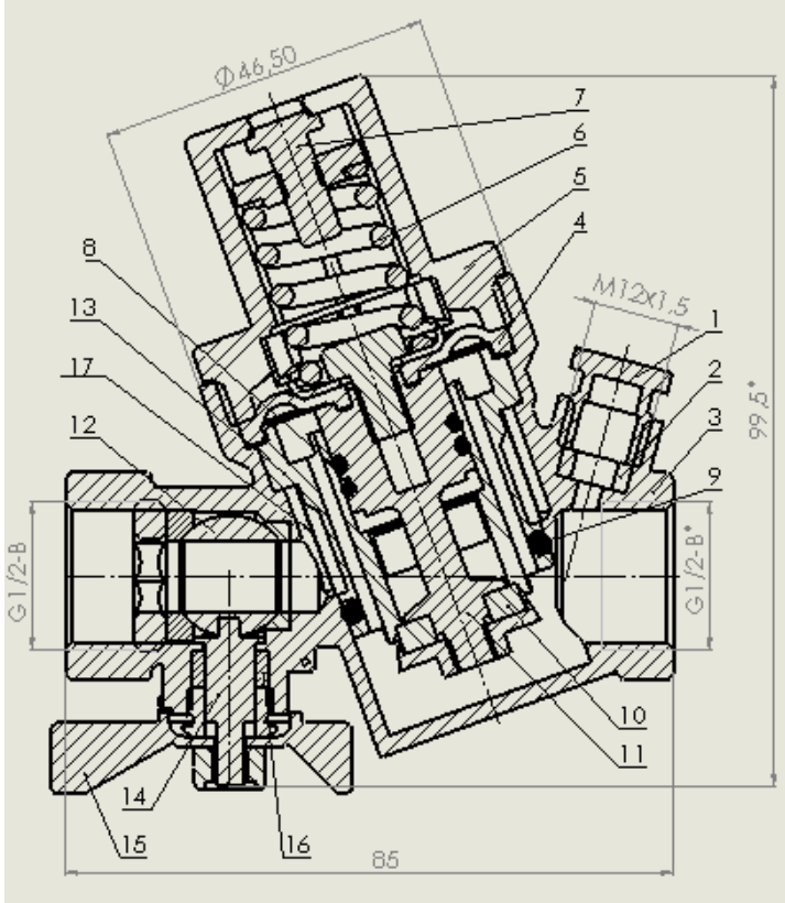
Рисунок 1 – Общий вид и габаритные размеры
