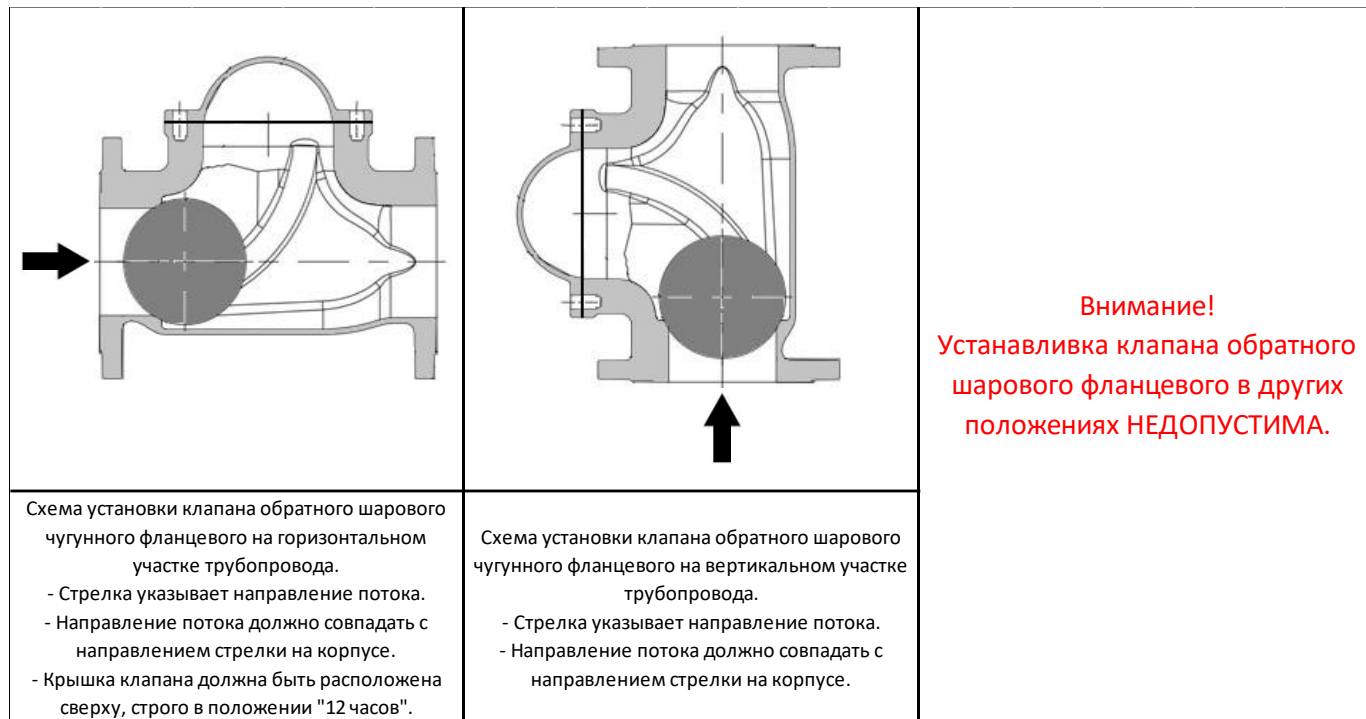
Схема №1 – Разрешенные положения установки клапана обратного шарового.
