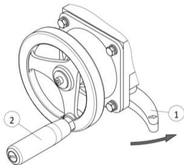
Рисунок 7 – Переключение на ручное управление
