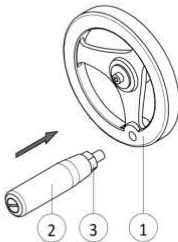
Рисунок 3 – Установка рукоятки 1 – Маховик, 2 – Рукоятка, 3 – Гайка
