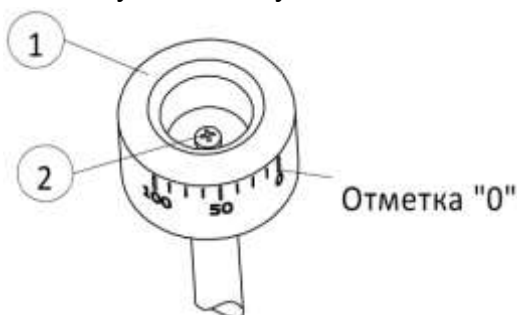
Рисунок 14 – Регулировка указателя положения
